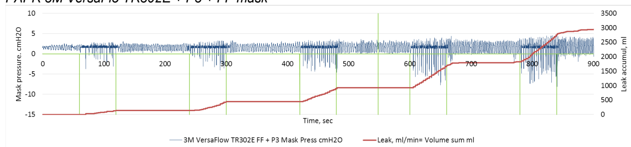
PAPR 3M VersaFlo TR302E + P3 + FF mask
